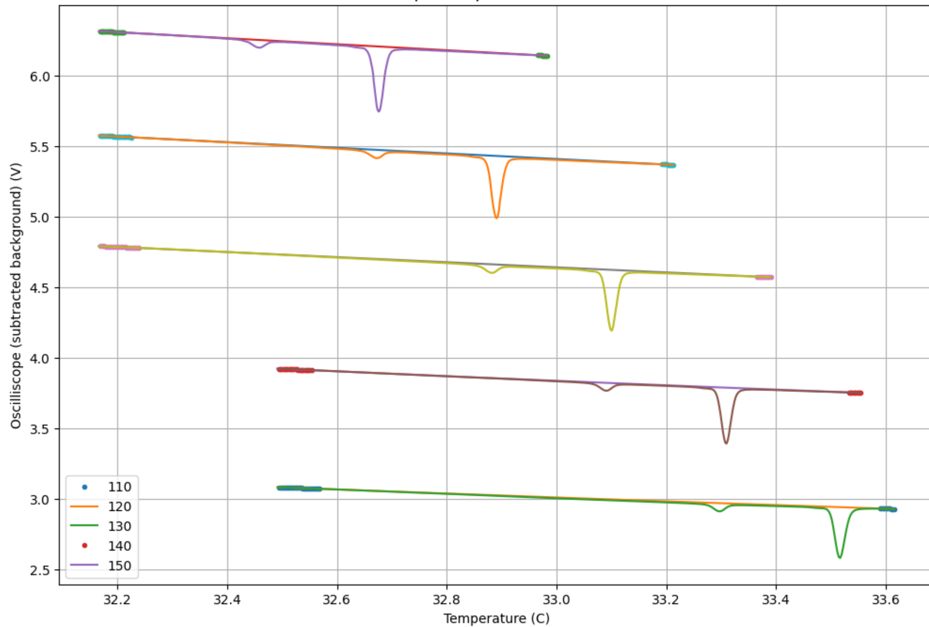
Absorption Dip (40 Celsius, lens)
