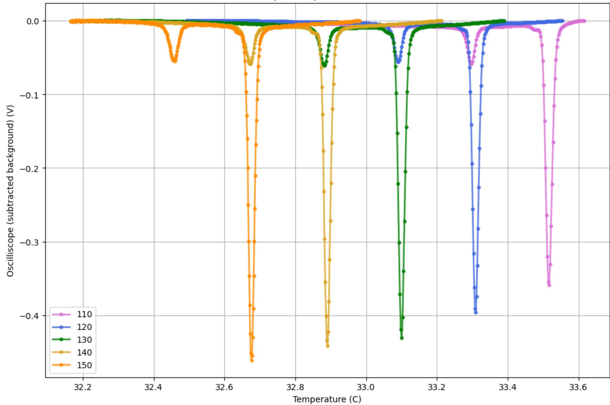
Absorption Dip (40 Celsius, lens)
